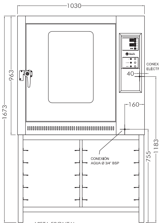
VISTA FRONTAL ESC. 1:16
