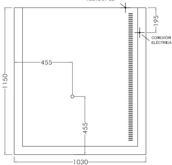
VISTA SUPERIOR
