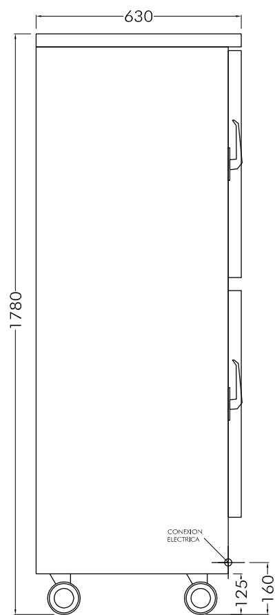
VISTA LATERAL ESC. 1:12
