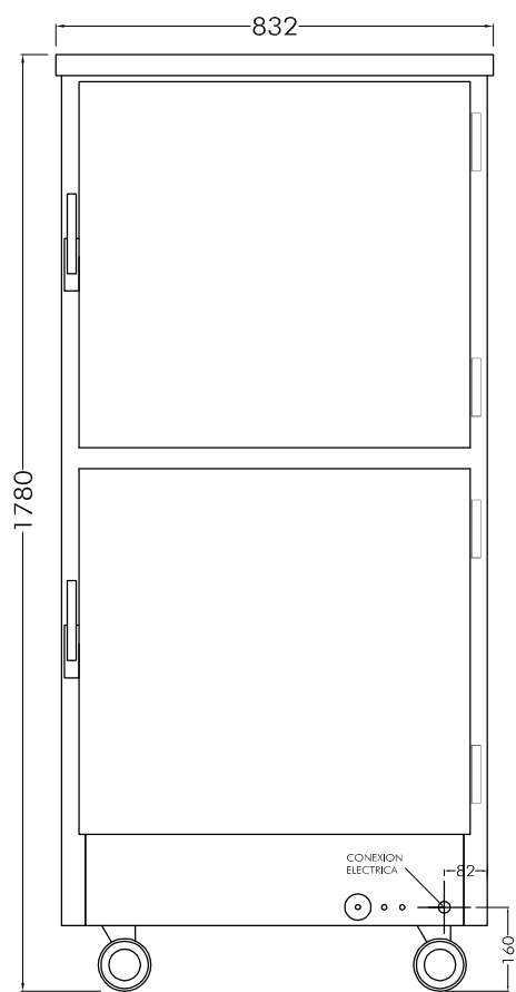
VISTA FRONTAL ESC. 1:12
