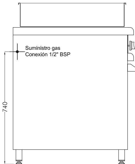
VISTA LATERAL ESC. 1:12
