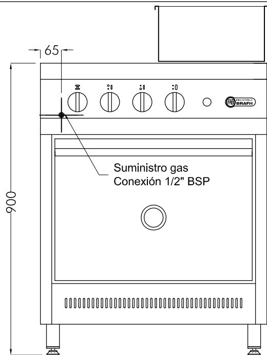
VISTA FRONTAL ESC. 1:12
