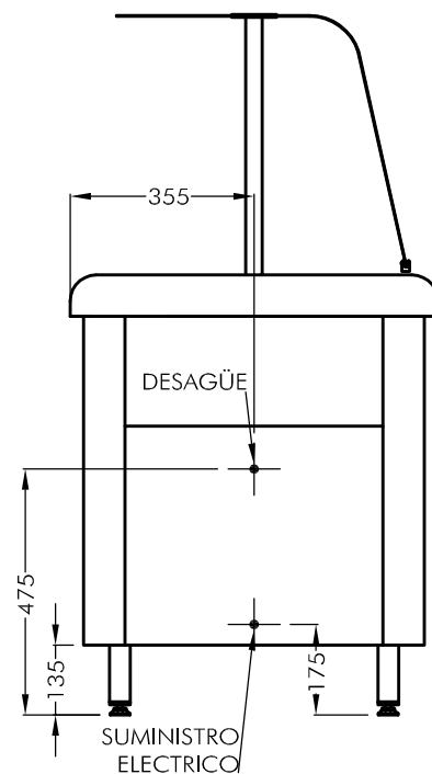
VISTA LATERAL ESC. 1:20
