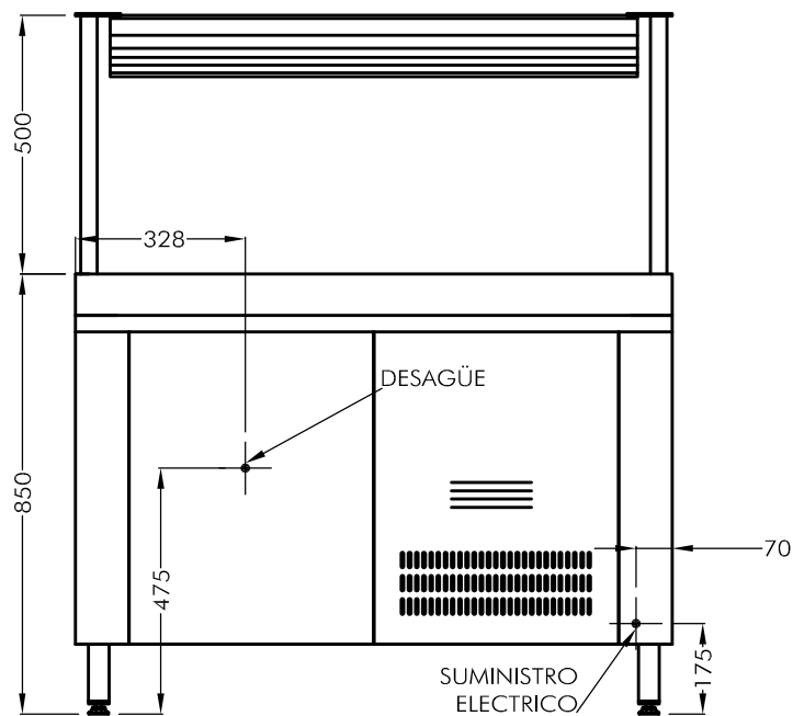
VISTA FRONTAL ESC. 1:20
