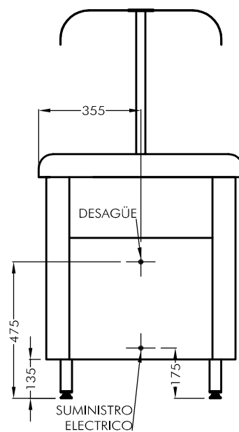
VISTA LATERAL ESC. 1:20
