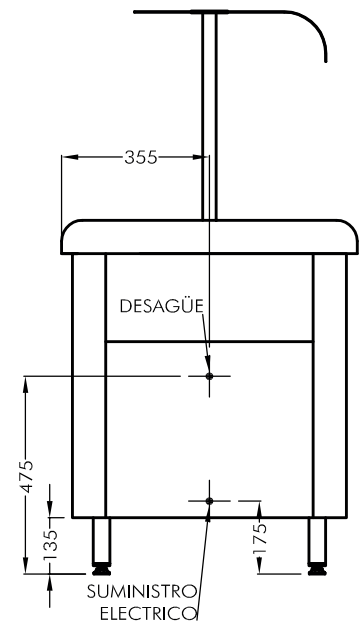
VISTA LATERAL ESC. 1:20
