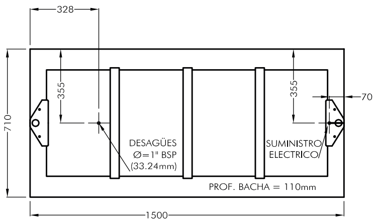
VISTA SUPERIOR ESC. 1:20
