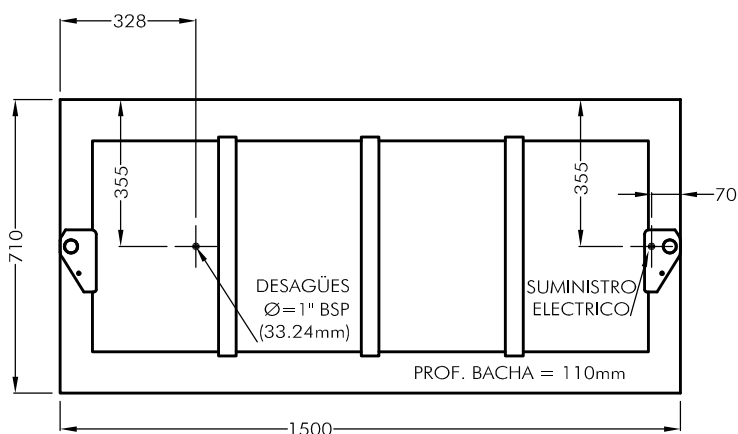
VISTA FRONTAL ESC. 1:20
