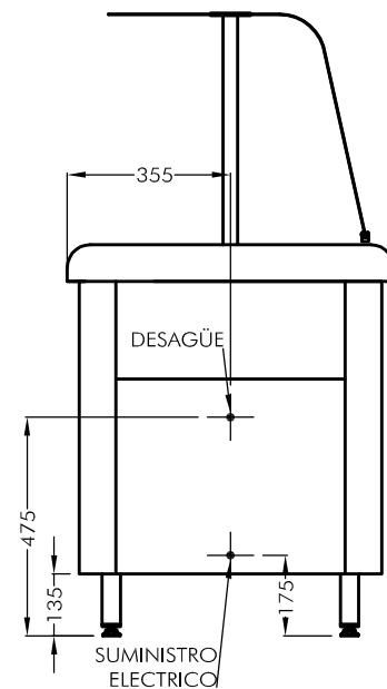
VISTA LATERAL ESC. 1:20
