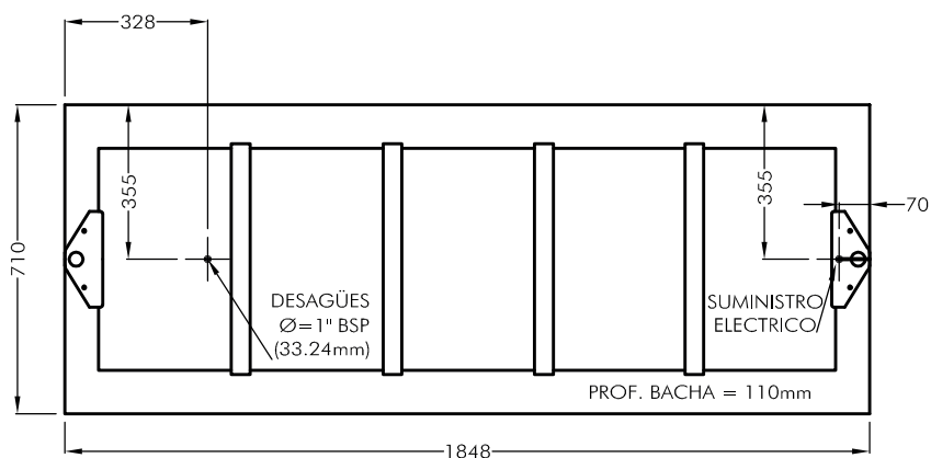
VISTA SUPERIOR ESC. 1:20
