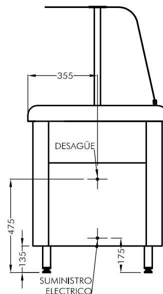
VISTA LATERAL ESC. 1:20
