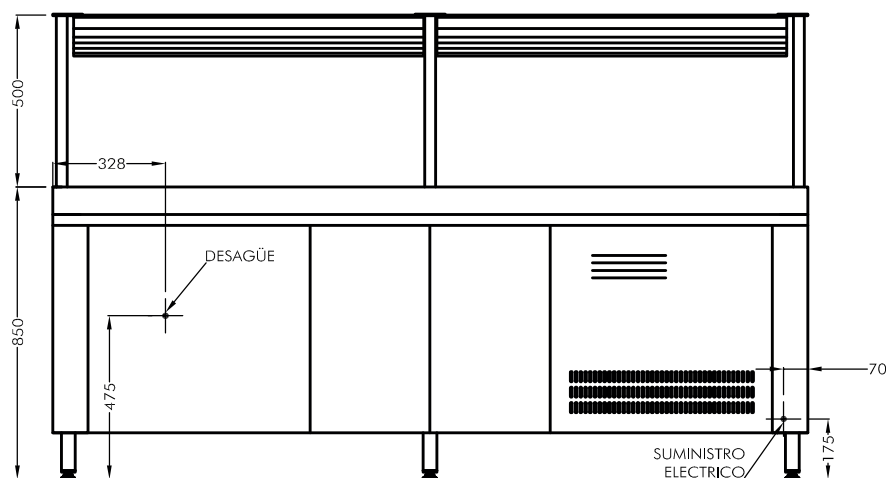
VISTA FRONTAL ESC. 1:20
