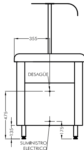
VISTA LATERAL ESC. 1:20
