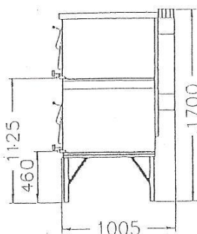
DIMENSIONES CAMARA COCCION
