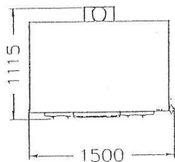
DIMENSIONES MAXIMAS
