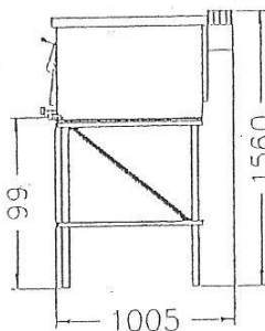
DIMENSIONES CAMARA COCCION
