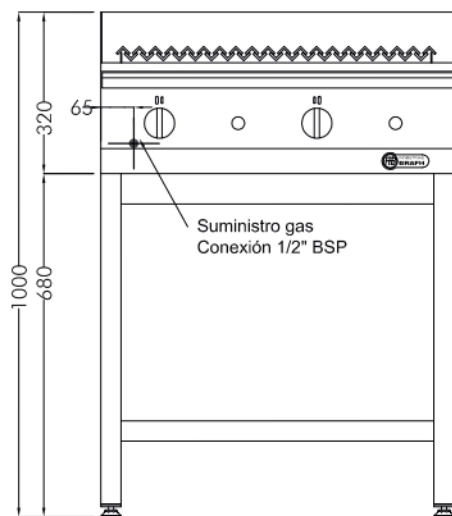
VISTA FRONTAL ESC. 1:15
