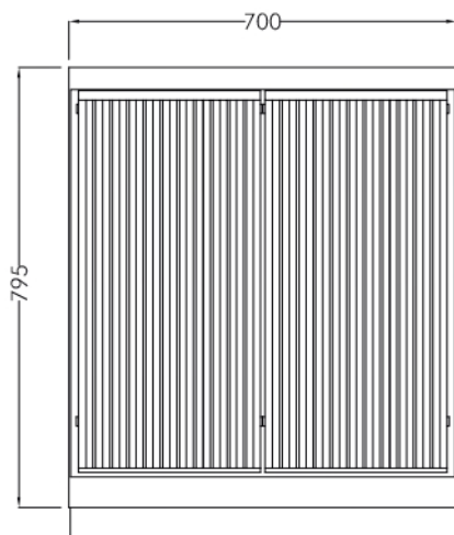
VISTA SUPERIOR ESC. 1:15
