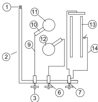
VISTA LATERAL ESC. 1:15
