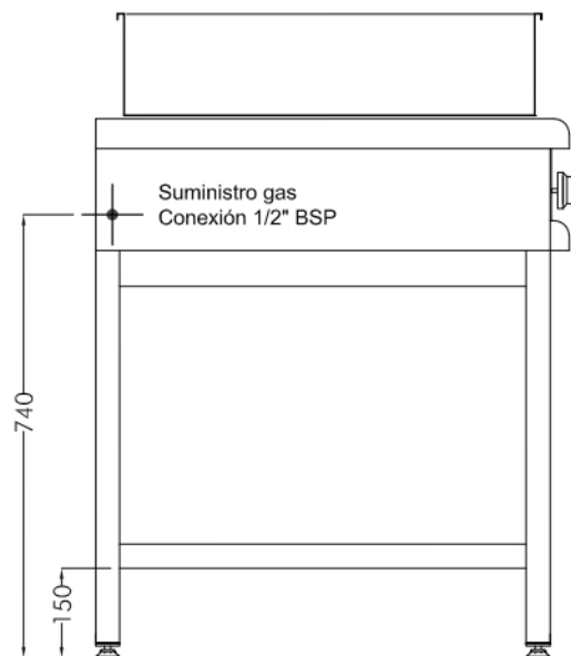
VISTA LATERAL ESC. 1:15
