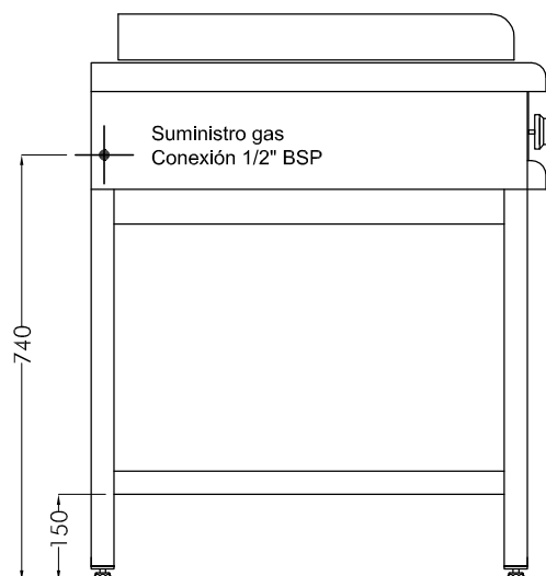
VISTA LATERAL ESC. 1:12
