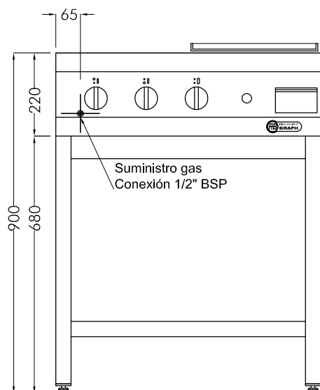
VISTA FRONTAL ESC. 1:15
