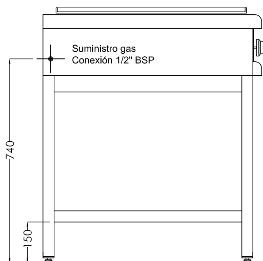
VISTA LATERAL ESC. 1:15
