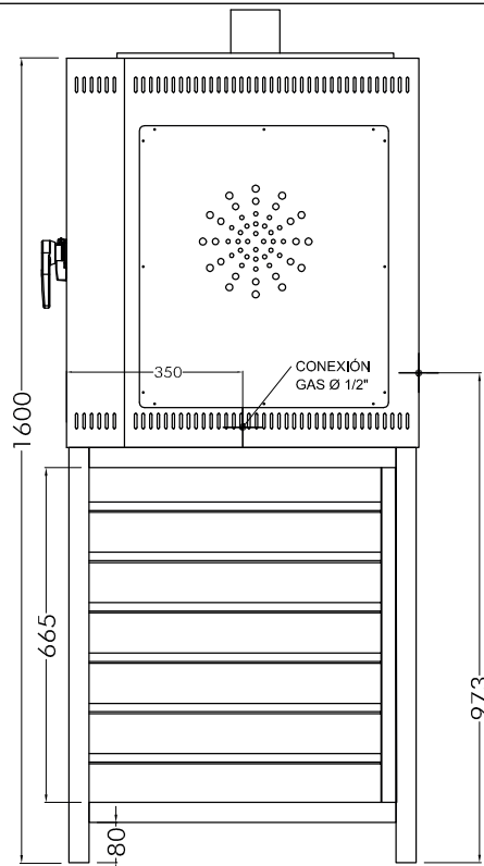
VISTA LATERAL ESC. 1:16
