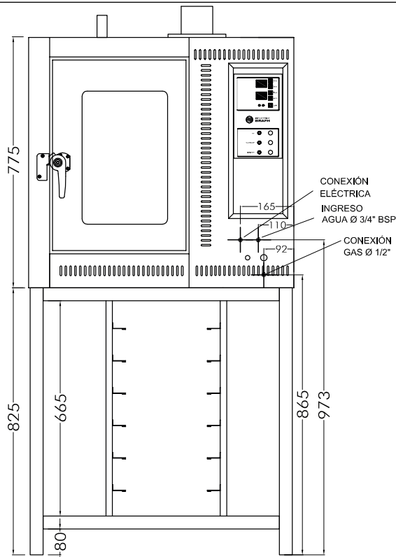
VISTA FRONTAL ESC. 1:16
